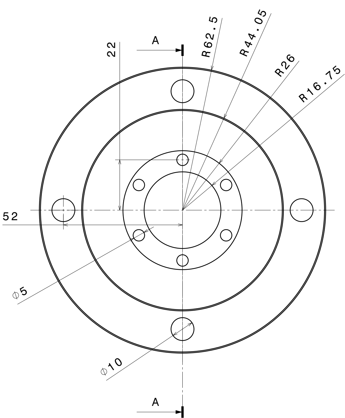
Vista frontale Scala: 1:1
